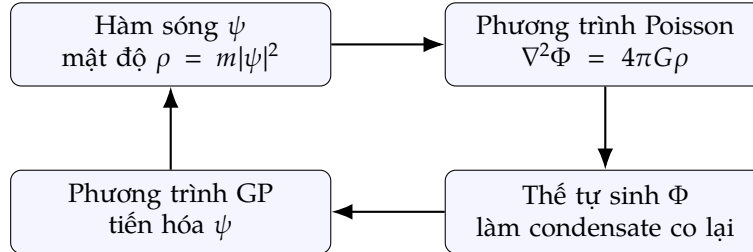
Hình 15: Vòng phản hồi tự nhất quán của hệ Gross–Pitaevskii–Poisson. Mật độ sinh ra thế hấp dẫn, còn thế hấp dẫn lại quyết định sự tiến hóa của chính mật độ ấy.
